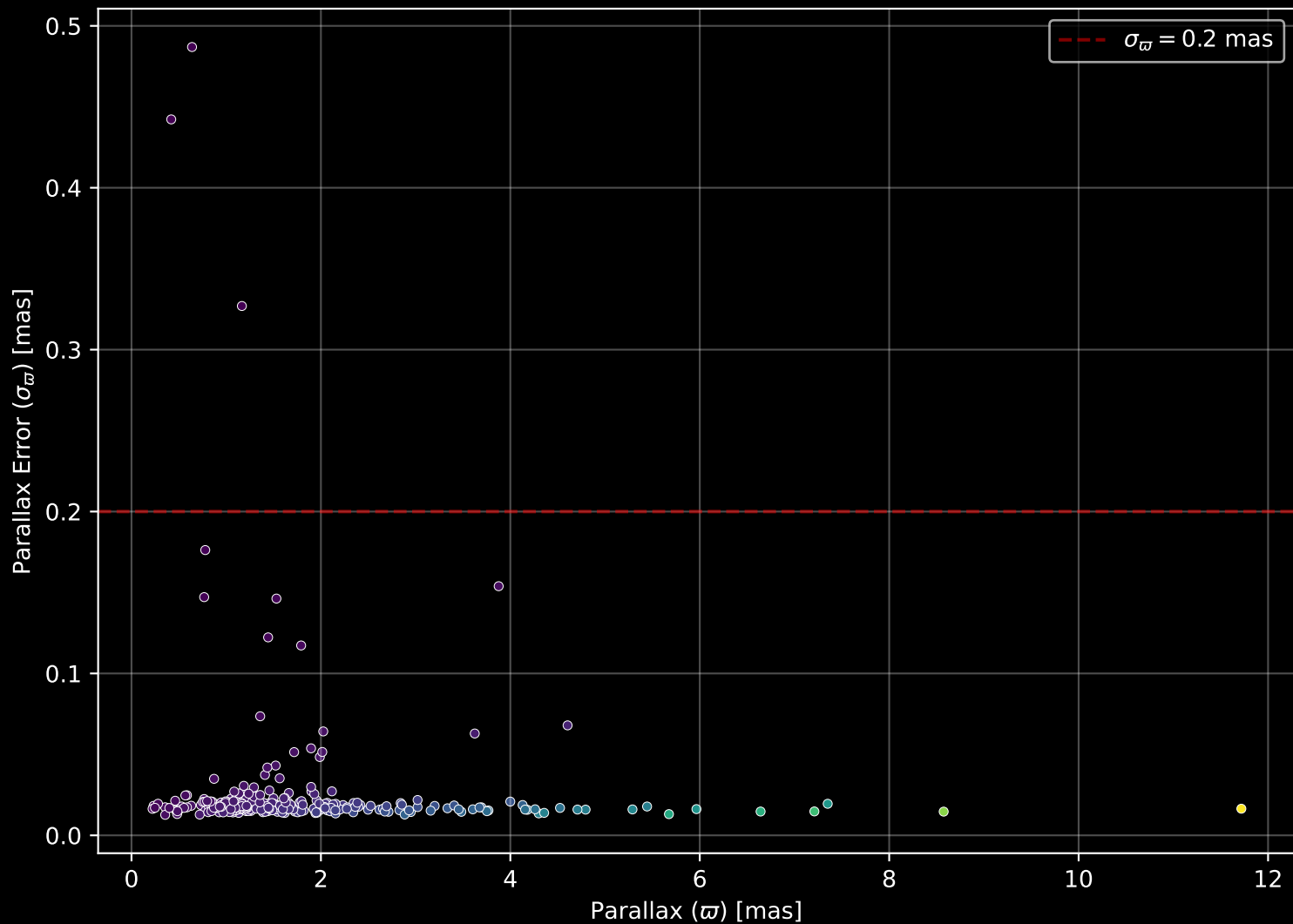
GALAH DR4 Field: [826] Parallax Quality (n= 281)
