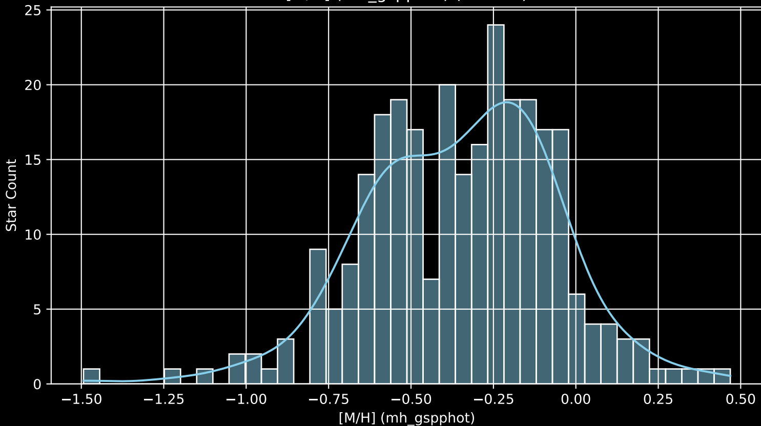
GALAH DR4 Field: [826] [M/H] (mh_gspphot) (n= 279)
