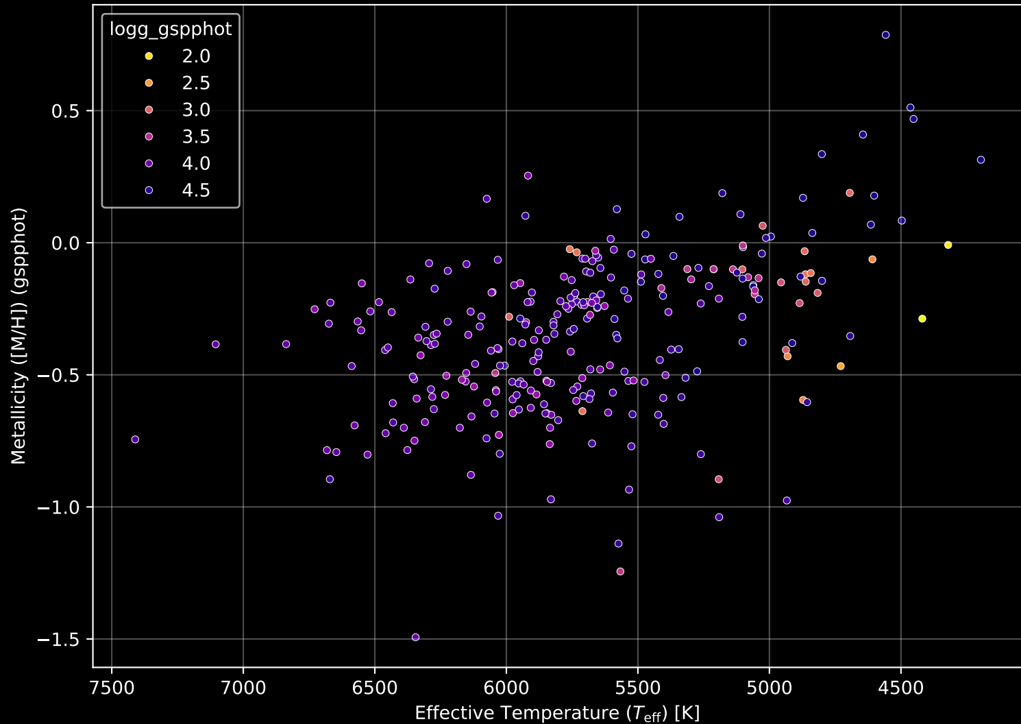
GALAH DR4 Field: [826] Stellar Population Parameters (n= 281)
