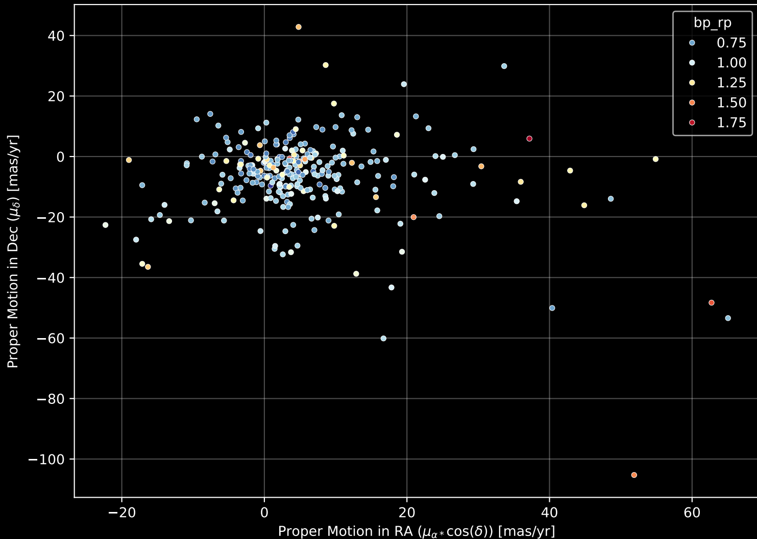
GALAH DR4 Field: [826] Proper Motion Diagram (n= 281)
